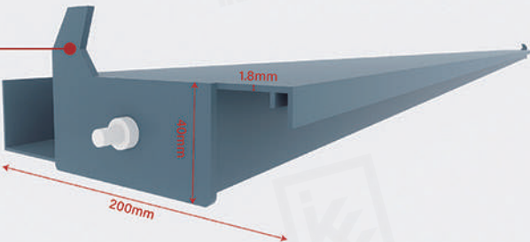
Blade : 200*40*1.8mm
