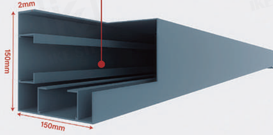
Post : 150*150*2.0mm
