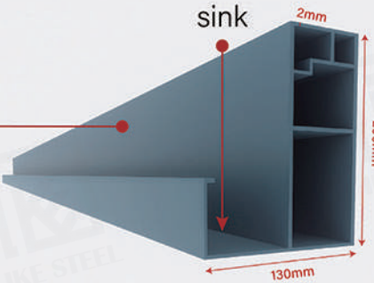
Frame : 200*130*2mm
