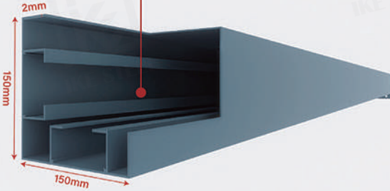
Post : 150*150*2.0mm
