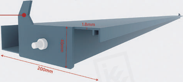
Blade : 200*40*1.8mm
