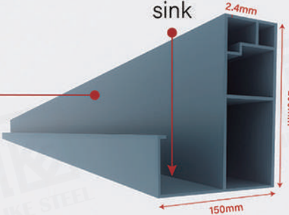
Frame : 200*150*2.4mm
